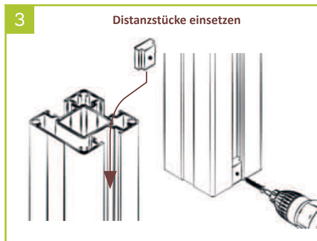
3 | Distanzstück hochkant in die Innenseite der Pfostennut einschieben, bündig mit der Unterkante des Pfostens abschließen, vorbohren und verschrauben.
