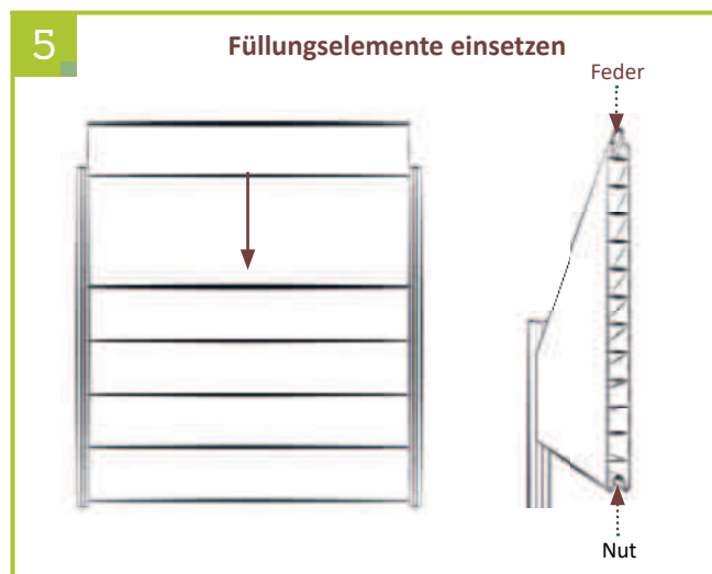
5 | Die Füllungselemente nacheinander von oben einschieben, dabei die Feder der Füllungselemente nach oben ausrichten.
