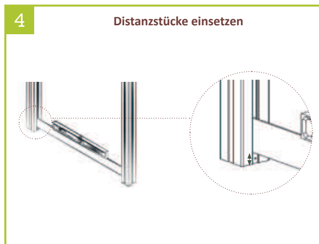
4 | Zuerst auf einer Seite das Distanzstück befestigen. Das Distanzstück der zweiten Seite mit Hilfe eines Füllungselementes und einer Wasserwaage ausrichten und befestigen.
