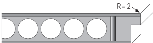
QUERSCHNITT TÜRLBLATT
